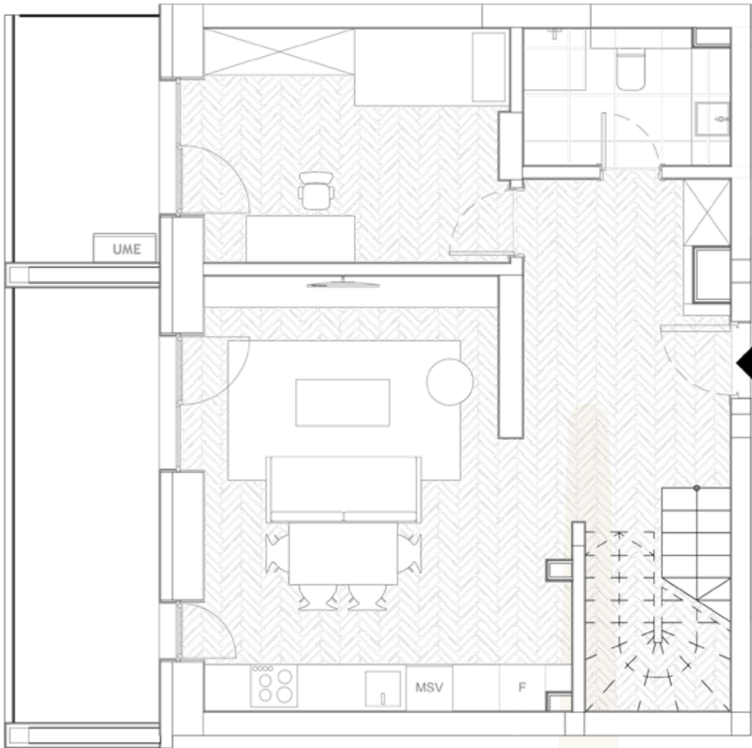
Plan etaj 11
